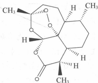
图1-2 青蒿素的结构
