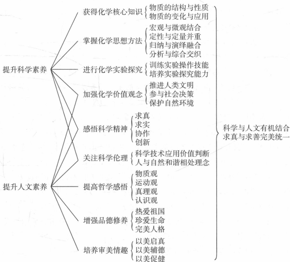
图 1-3 中学化学学科的育人价值框架结构
