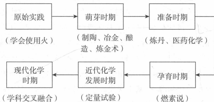
图 1-1 化学科学体系的形成和发展过程
