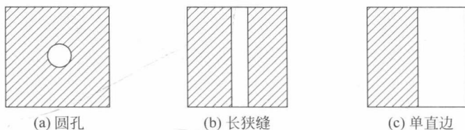
图 1.1.1 典型的衍射屏
