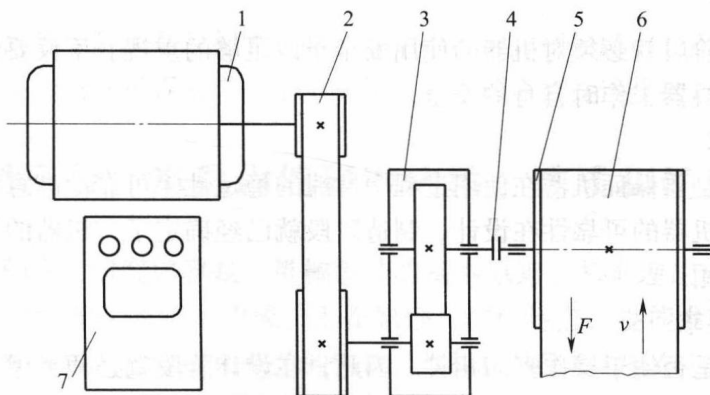
图 0-4 带式输送机
