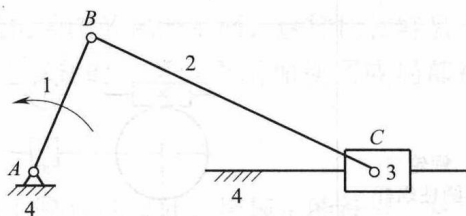
图 1-4 曲柄滑块机构
