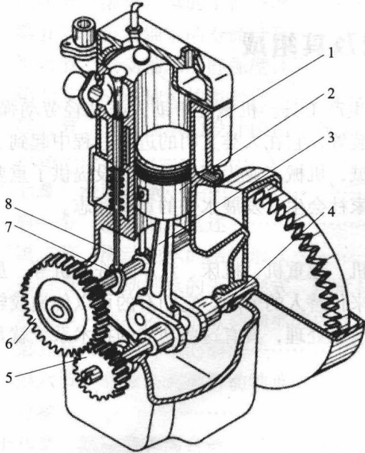
图 0-1 内燃机
