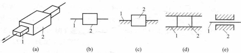
图 1-2 移动副及其表示方式
