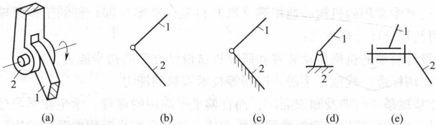
图 1-1 转动副及其表示方式
