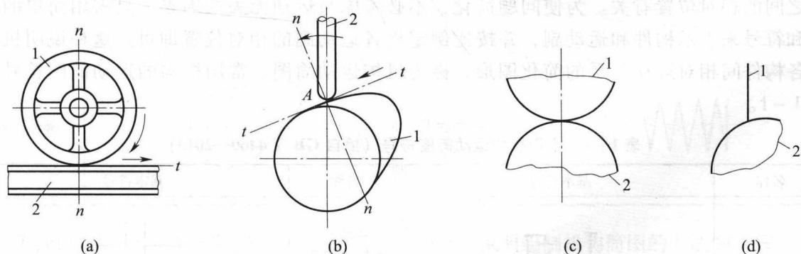
图 1-3 高副的表达方式
