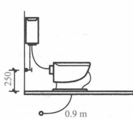
图 1-3 坐式大便器
