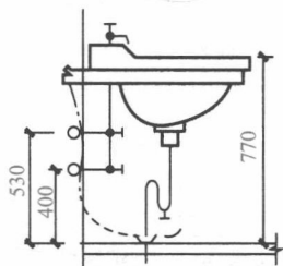
图 1-1 洗脸盆
