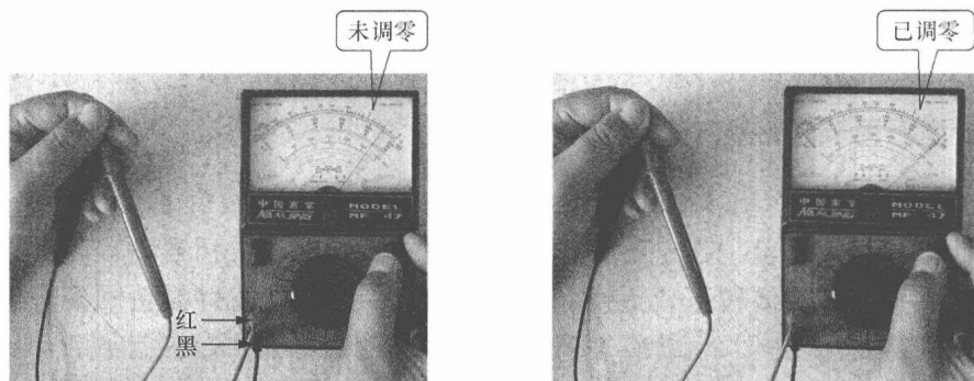
图 1-6 指针型万用表表针调“0”示意图
