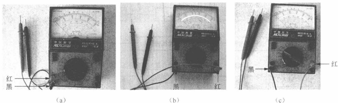
图 1-5 指针型万用表安装表笔示意图
