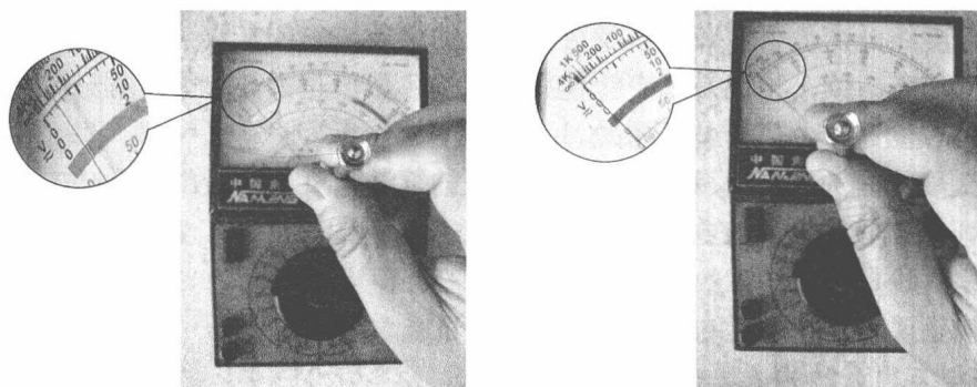
图 1-4 指针型万用表表针复位的调整
