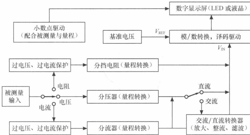
图 1-3 数字型万用表的组成框图
