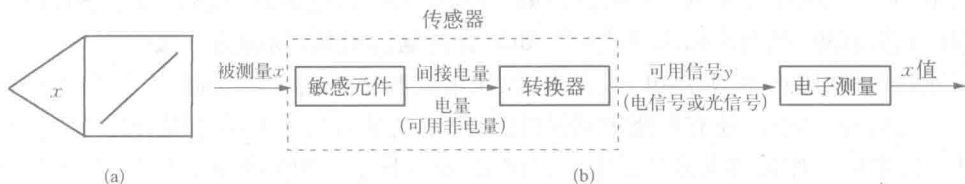
图 1.1 传感器组成
