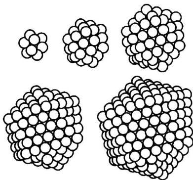
图 1.3 原子数为 13, 55, 147, 309, 561...的稳定态氩原子簇示意图
