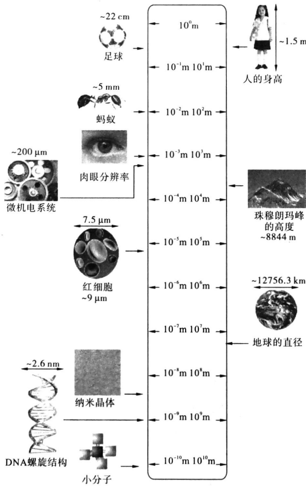
图 1.2 不同尺度的物质：微米到纳米
