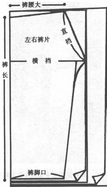
图 1-8 中式长裤裁剪示意图
