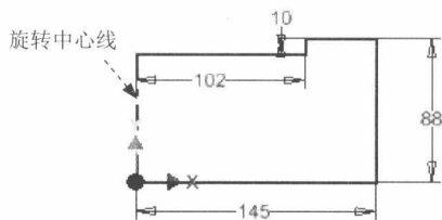
图 1.3 截面草图
