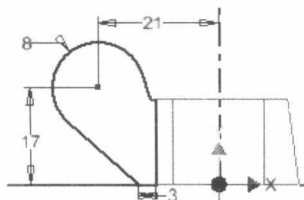
图 2.5 截面草图
