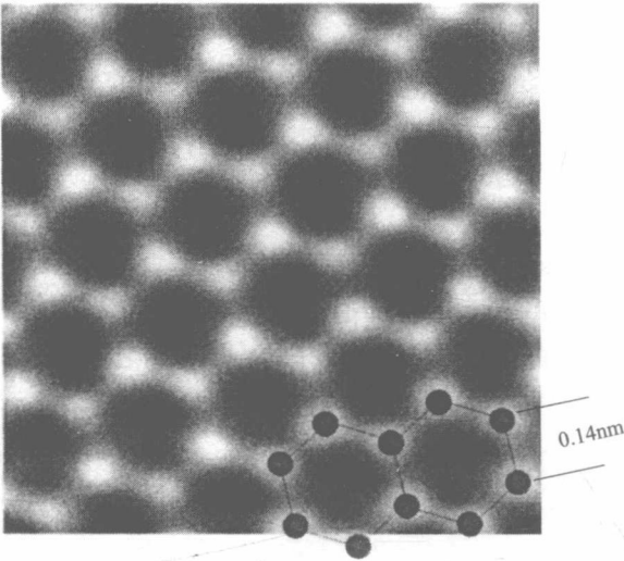
图 1.8 高质量石墨烯的 HRTEM 像
