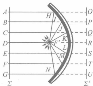
图 1-5 抛物面成像示意图
