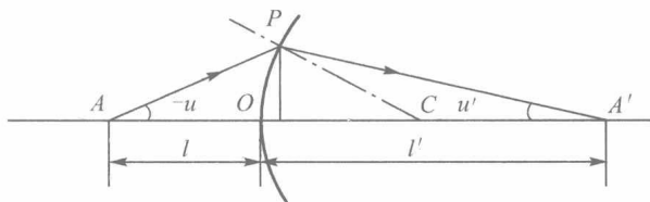
图 2-2 近轴光路计算
