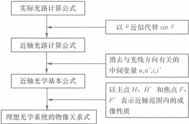
图 2-1 物像关系计算示意图
