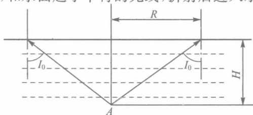
图1-4 游泳者水中仰视天空示意图
