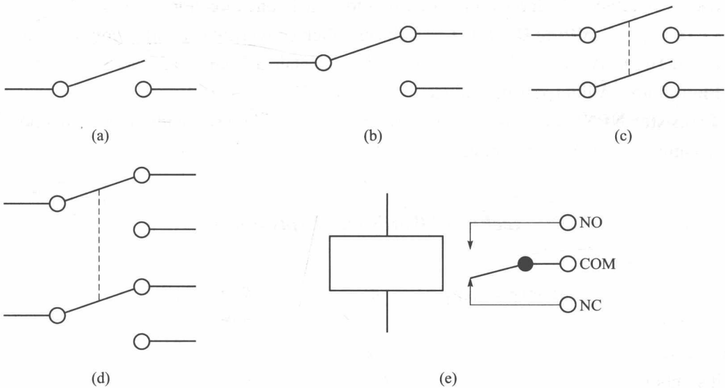
Fig. 1-7 Switches (a) SPST; (b) SPDT; (c) DPST; (d) DPDT; (e) Relay
