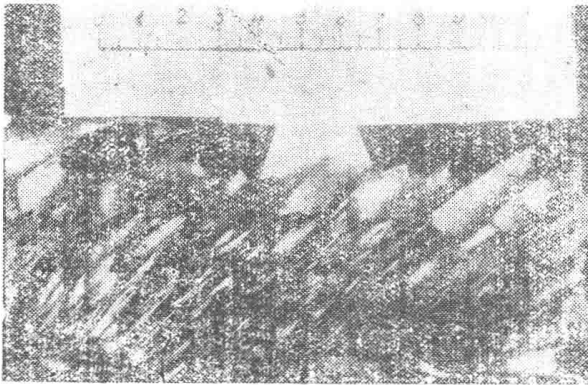
图5 典型的鱼鳞状破坏图。
