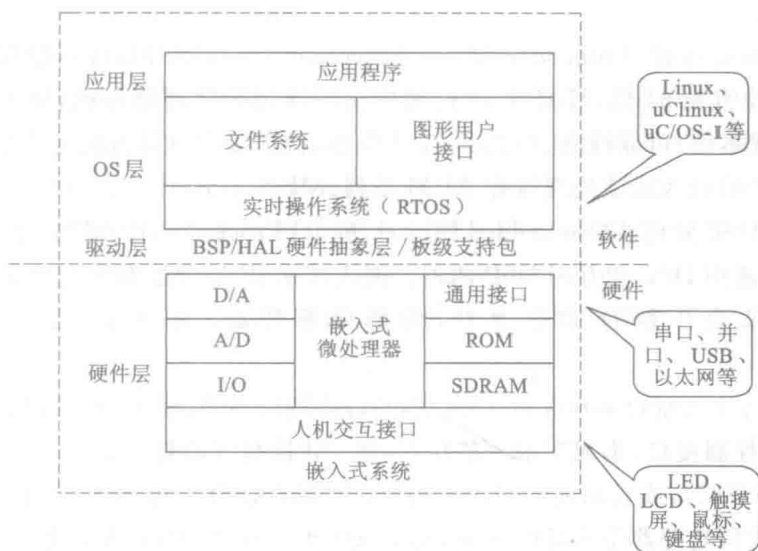
图 1-1 嵌入式系统组成
