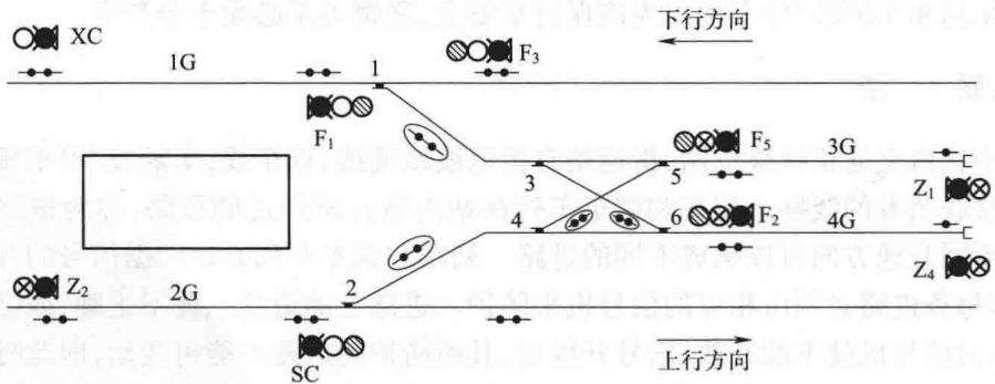
图 1-1 某折返站的信号设备平面布置图
