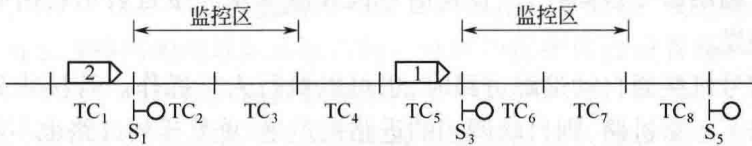
图 1-4 多列车进路示意图
