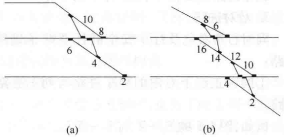
图 1-3 三动道岔和四动道岔
