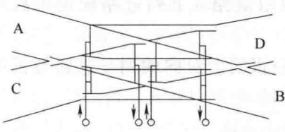
图 1-2 复式交分道岔
