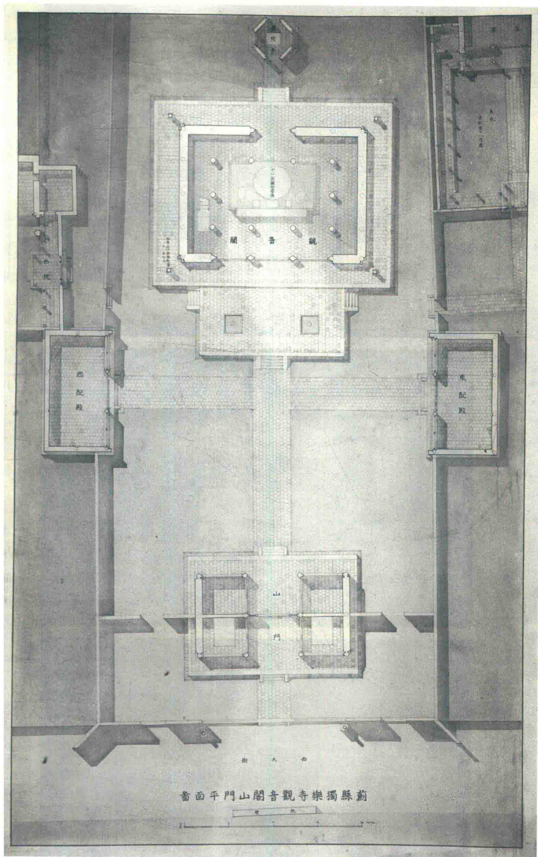
图2-1-8 薊县独乐寺观音阁、山门平面图(莫宗江绘)
