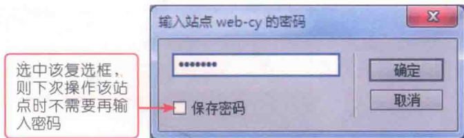
图1-43 设置密码
