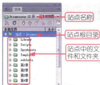
图 1-24 “文件”面板
