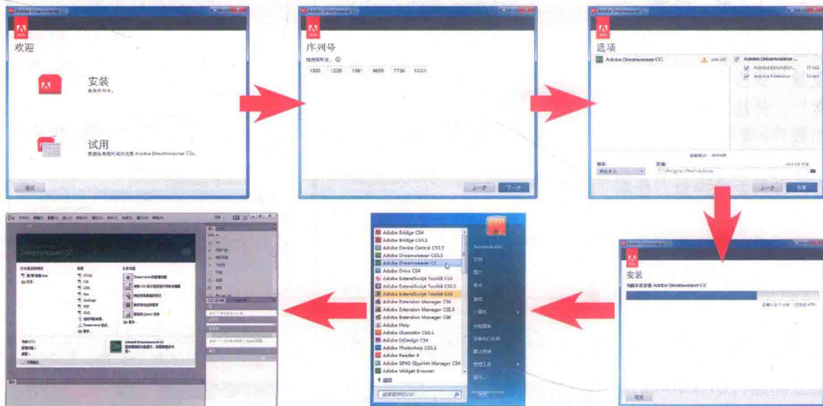
图1-1 操作流程
