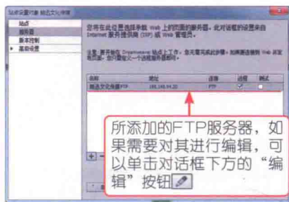
图1-33 “服务器”选项
