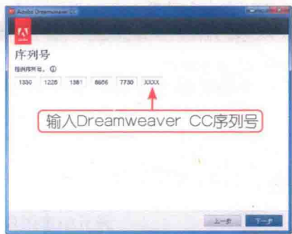
图1-5 输入序列号
