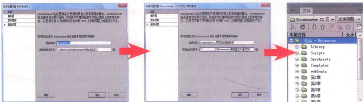
图 1-20 操作流程
