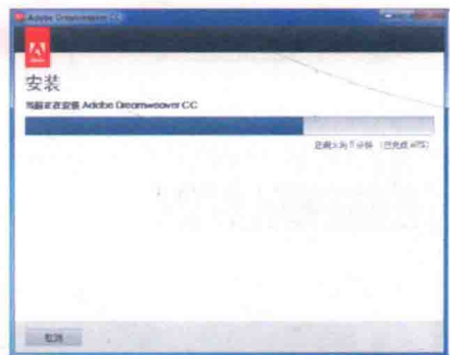
图1-7 安装界面
