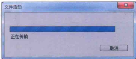
图1-44 同步文件
