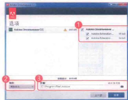
图1-6 选项界面
