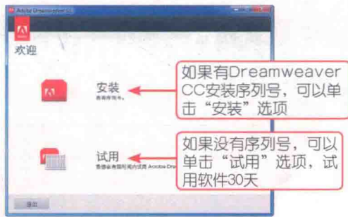
图1-3 欢迎界面
