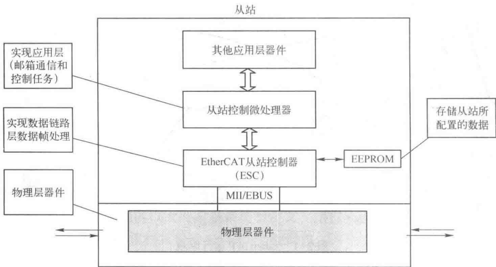
图 2-3 EtherCAT 从站组成
