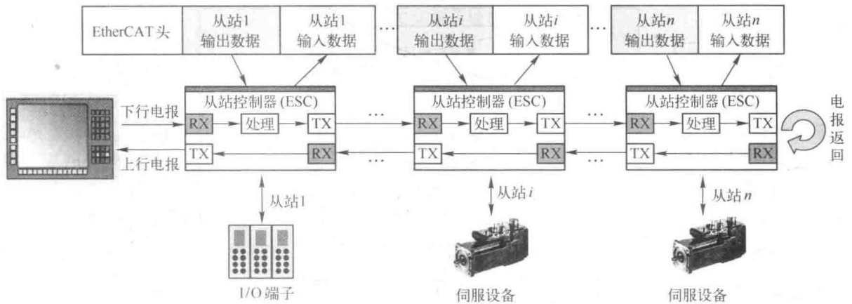
图 2-1 EtherCAT 运行原理
