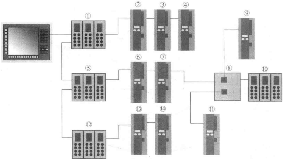
图 2-5 EtherCAT 线形拓扑结构
