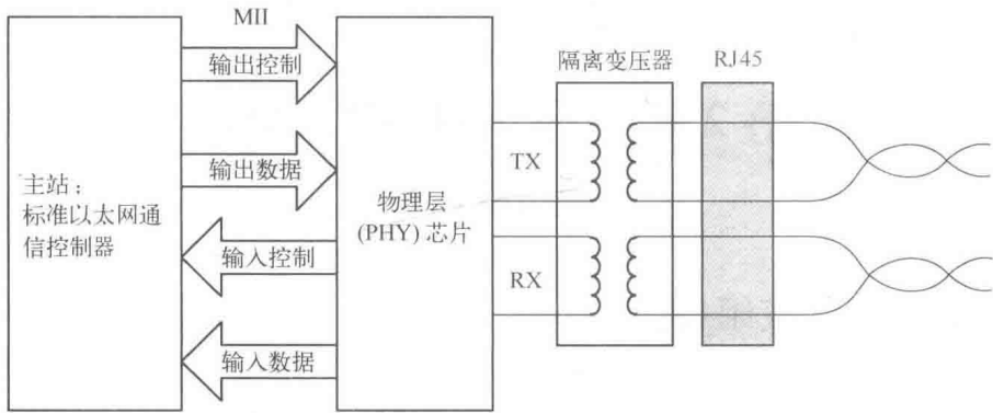
图 2-2 EtherCAT 物理层连接原理图
