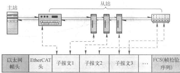
图 1-2 EtherCAT 运行原理
