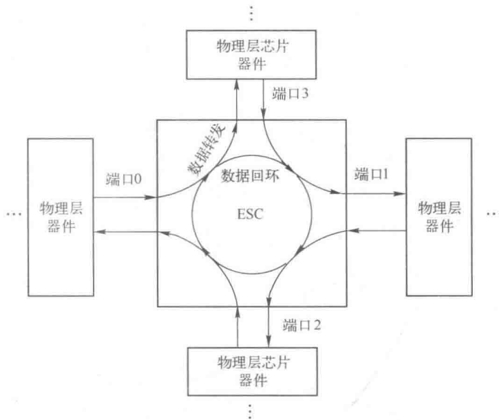
图 2-4 ESC 数据传输顺序
