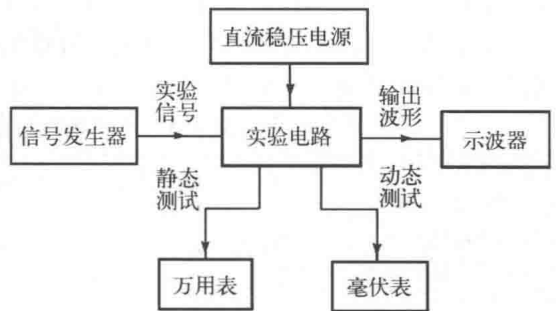
图1-1 电子技术实验中测量仪器连接图
