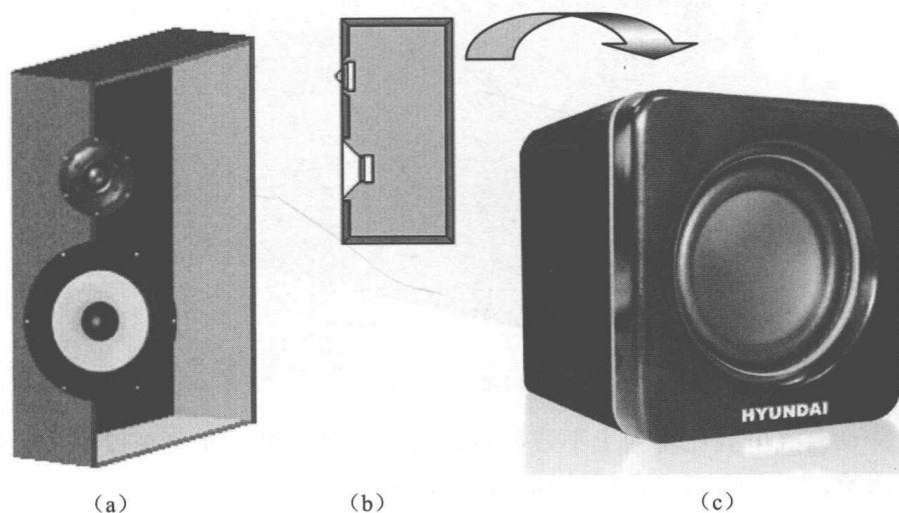
图 1-7 密闭式音箱
