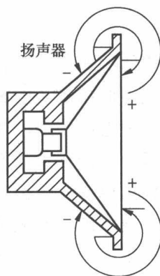
图 1-2 扬声器发声时的示意图
