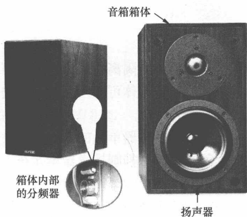
图 1-1 音箱的构成
