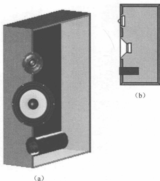
图 1-8 倒相式音箱结构图
