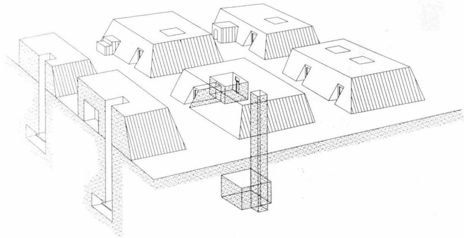
1.1.1.1 玛斯塔巴轴测图
