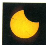
partial eclipse 日偏食
