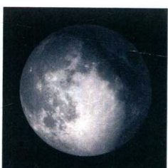
waning gibbous 亏凸月
