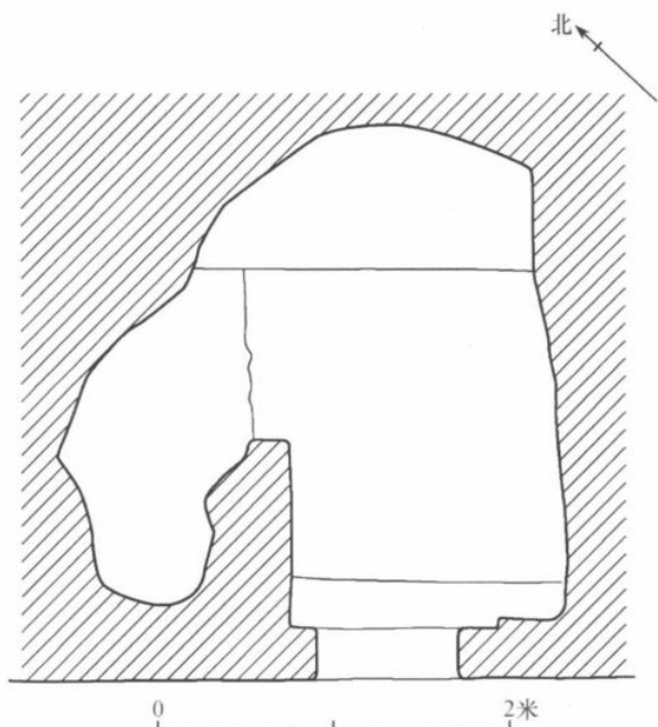
图15 第3窟平面图
