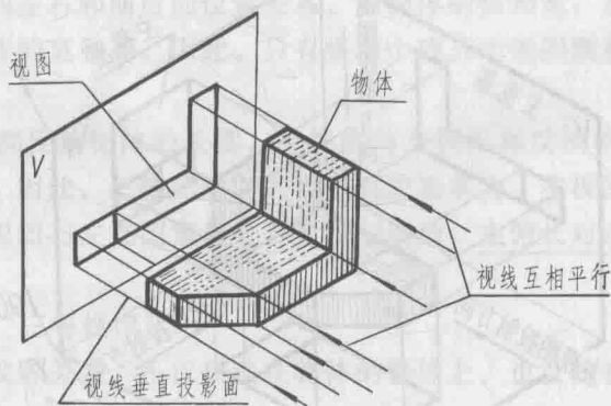
图 1-10 视图的概念
