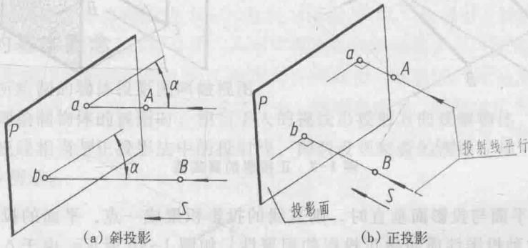
图 1-3 斜投影和正投影
