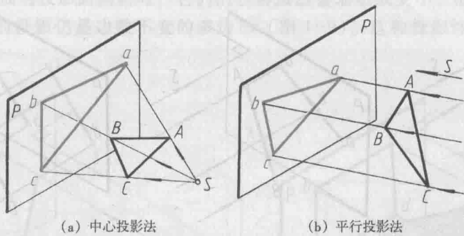
图 1-2 两种投影法
