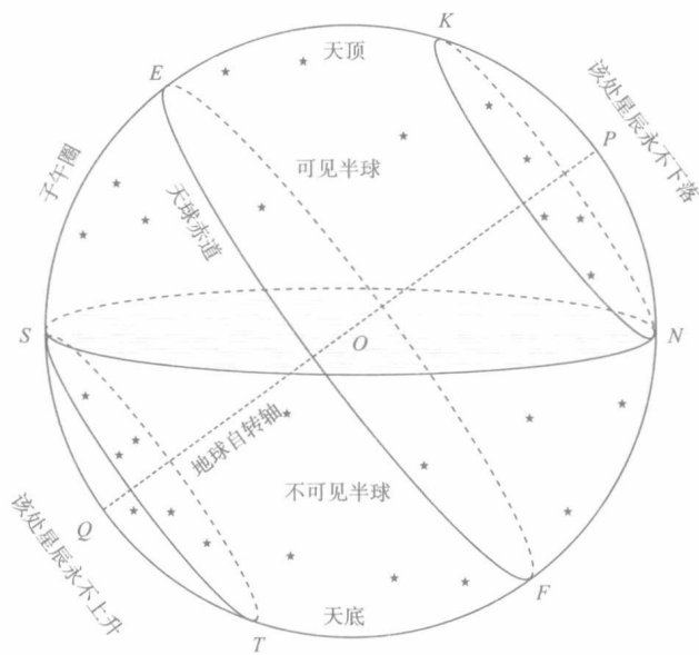
图1 我们眼中的天球
