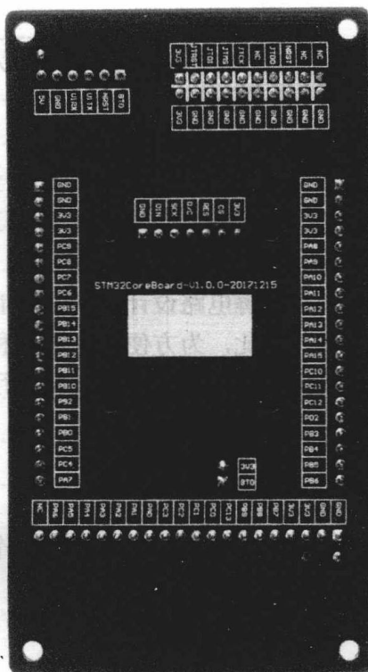
图 1-2 STM32 核心板背面
