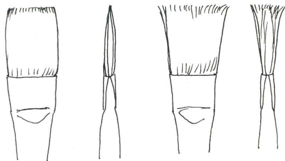
优质猪鬃毛画笔（左）从侧面看笔尖逐渐变窄。劣质猪鬃毛画笔（右）像一个小笤帚似的散开。
