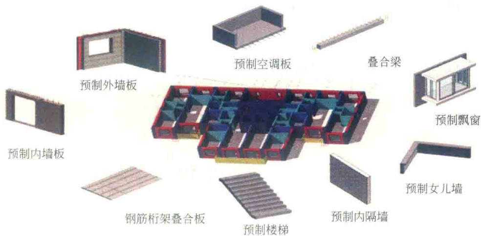
图 1-1 装配式剪力墙结构体系预制构件示意
