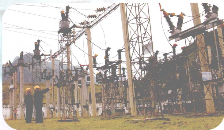
变电站
