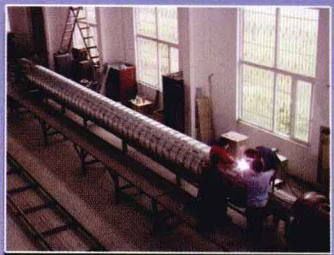
高压绕管式换热器
