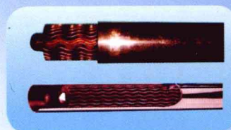
内翅片换热管
