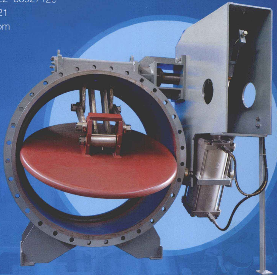
分子筛纯化系统用三杆阀
