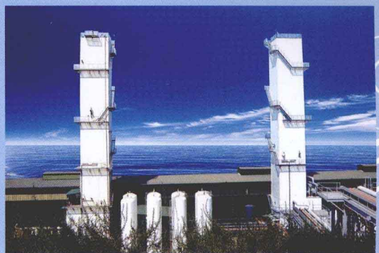
出口土耳其2 × 10000 m 3 /h空分设备
