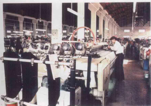
高速剑杆机织造车间
