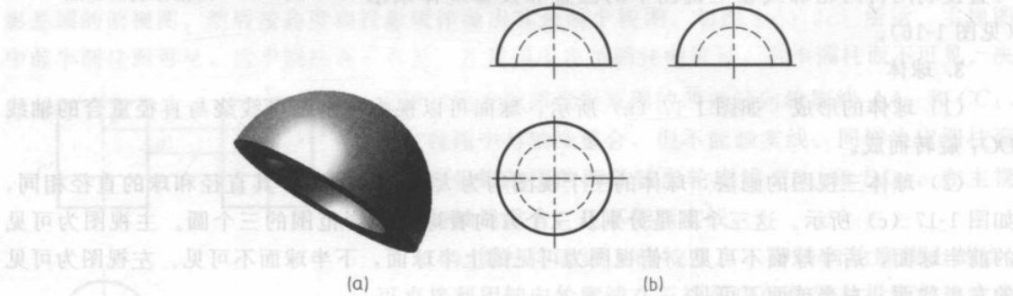
图 1-20 球形封头及其三视图
