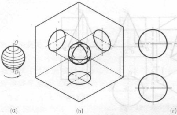
图 1-17 球的三视图
