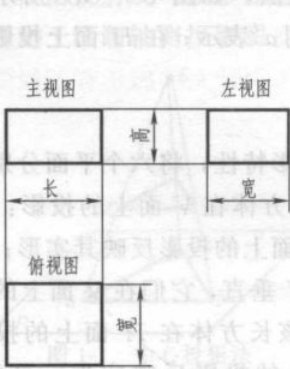
图 1-8 三视图度量关系
