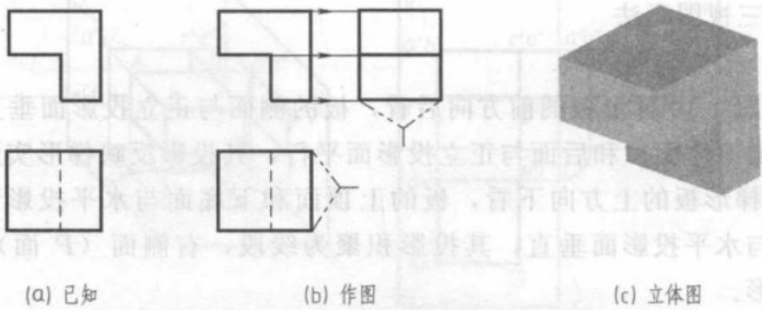
图 1-12 画出平面立体的左视图
