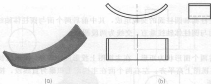
图 1-21 鞍形板及其三视图
