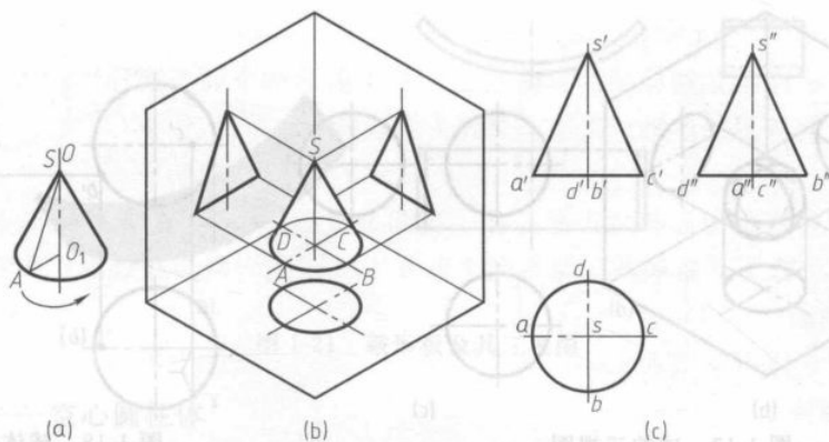
图 1-15 圆锥的三视图
