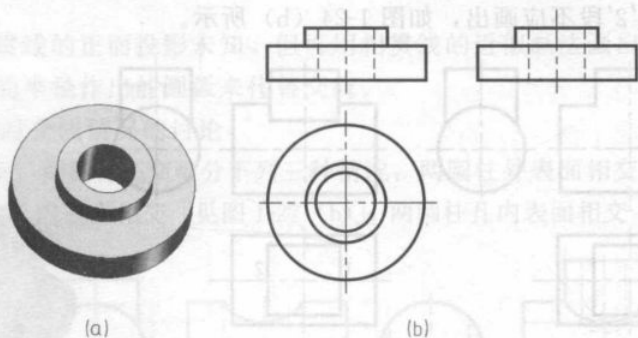
图 1-22 法兰板及其三视图
