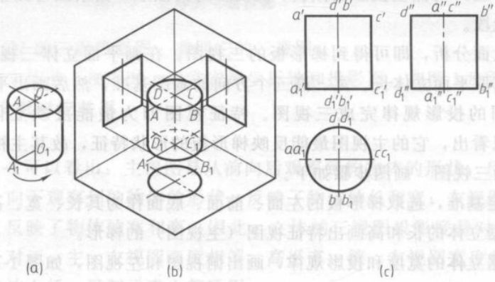
图 1-13 圆柱体的三视图
