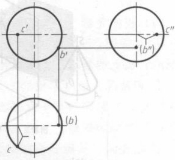
图 1-18 球体表面取点
