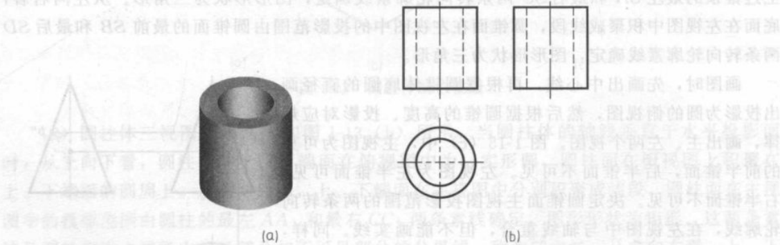
图 1-19 筒体及其三视图
