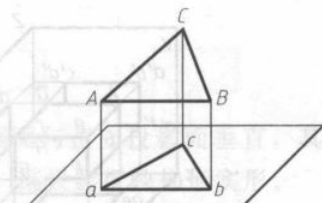
图 1-6 正投影特性四
