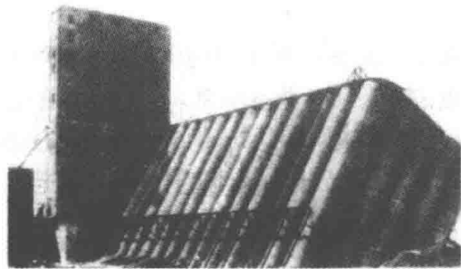
图 0.2 加拿大谷仓因地基强度不足而倾斜
