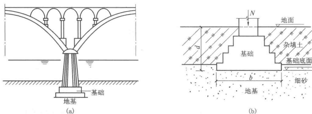
图 0.1 地基与基础
