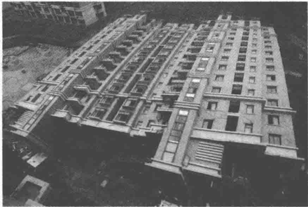
图 0.3 上海莲花景苑整体倒塌
