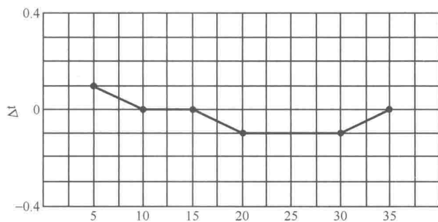
图 2-2 温度计的校正曲线( ^{\circ}\text{C} )
