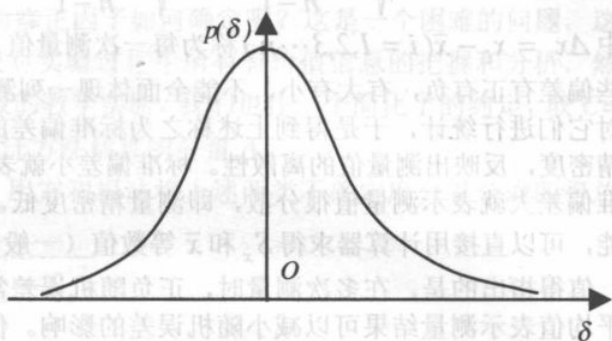
横坐标表示绝对误差,纵坐标表示某误差出现的概率
