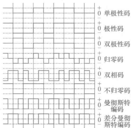
图 1.2 常用编码方案
