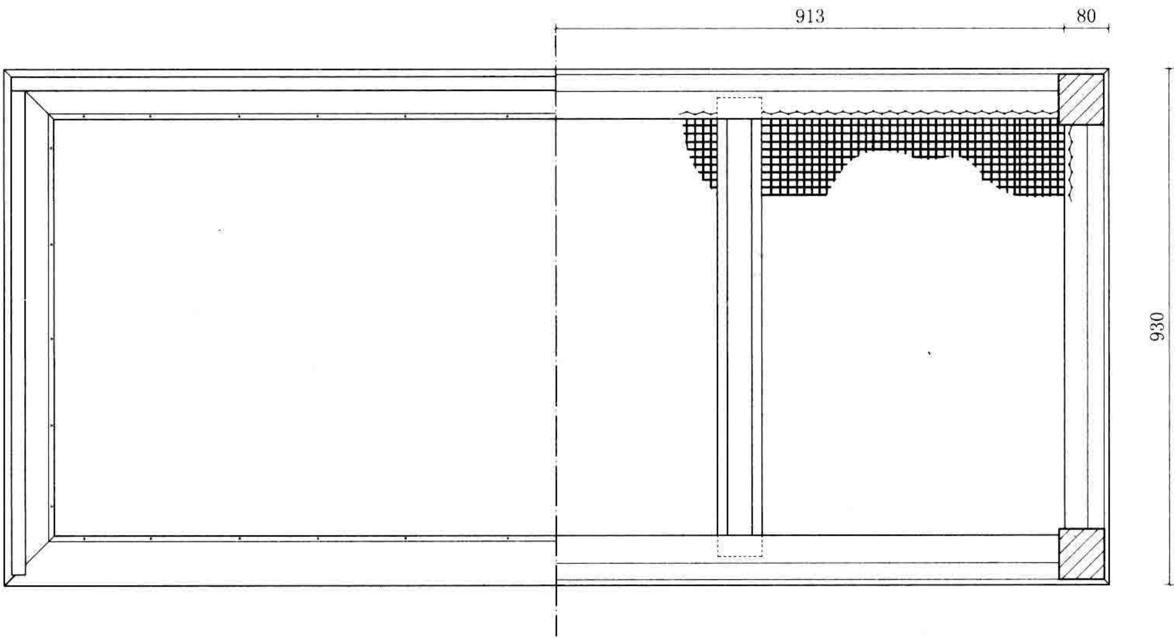
俯视图
