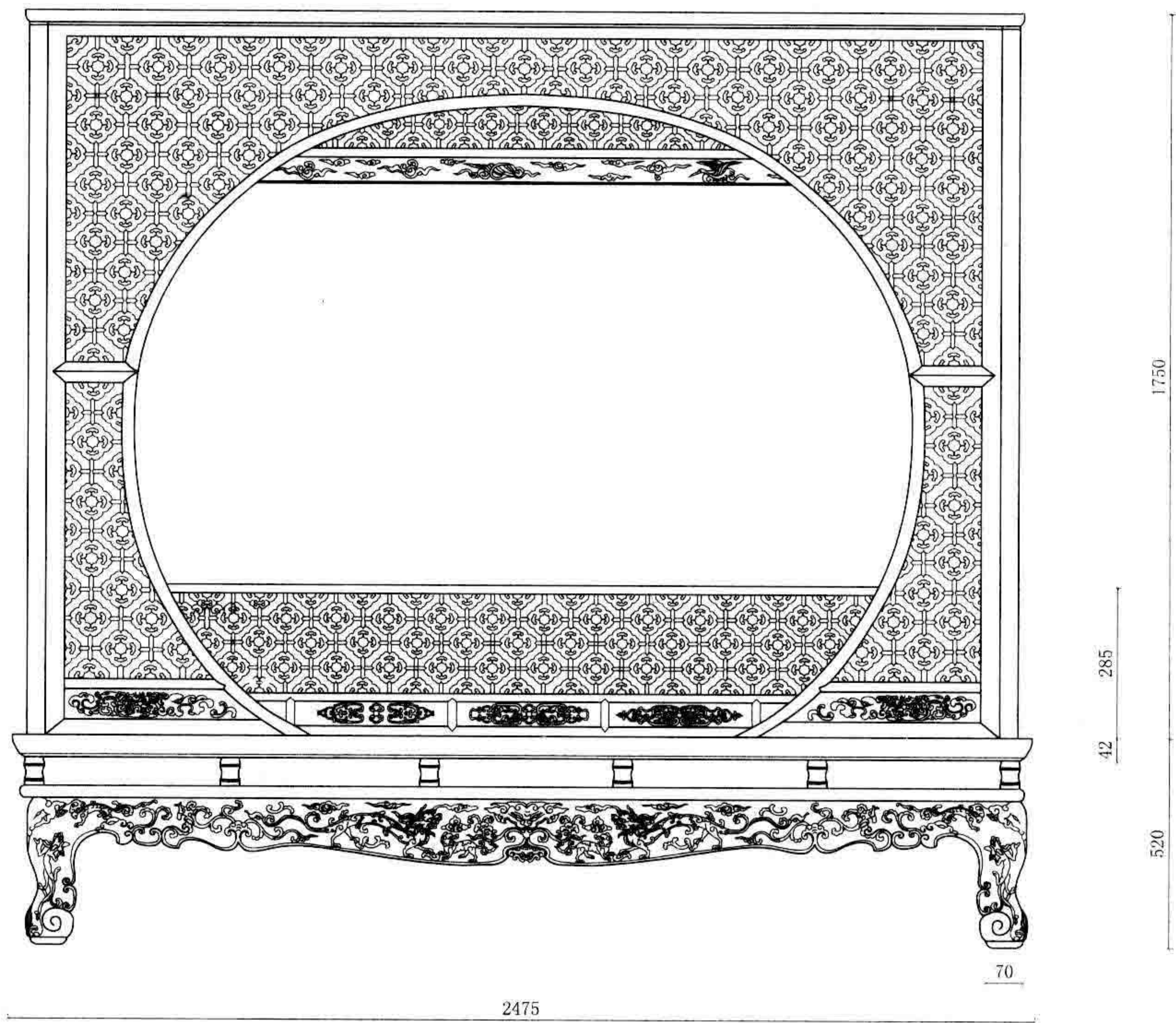
主视图
