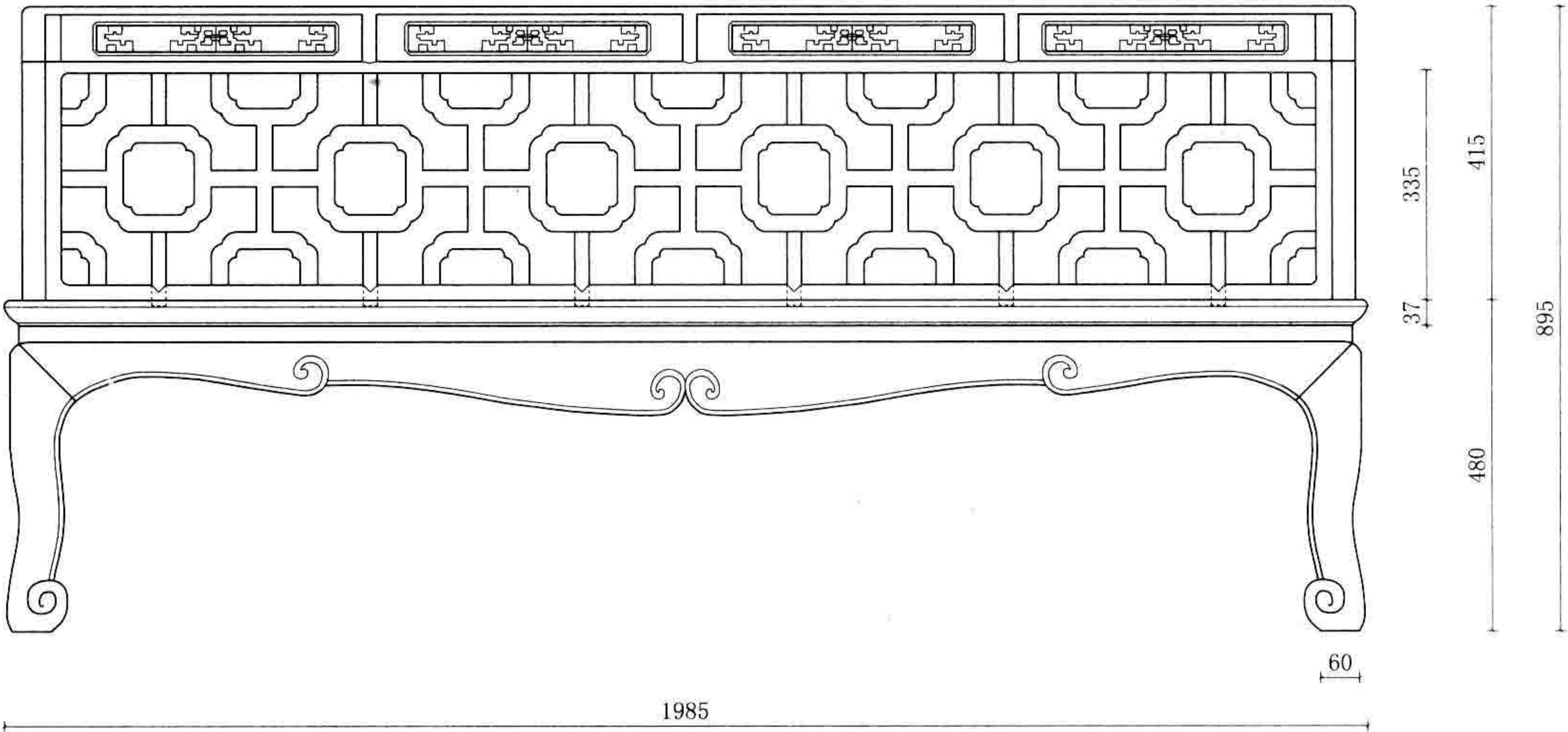
主视图
