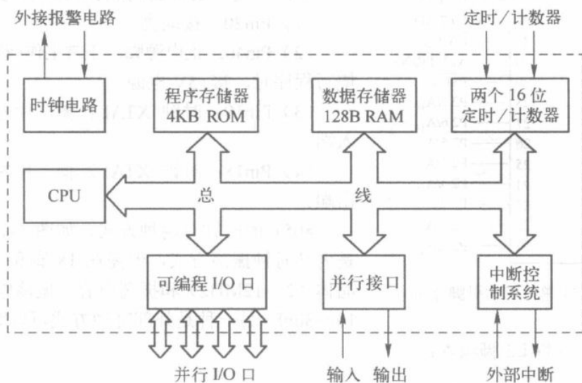
图 1-1-1 MCS-51 系列单片机的内部结构示意图
