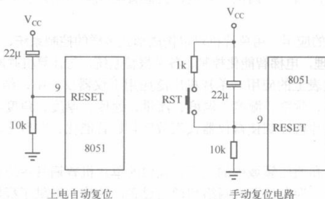
图 1-1-4 MCS-51 单片机的复位电路
