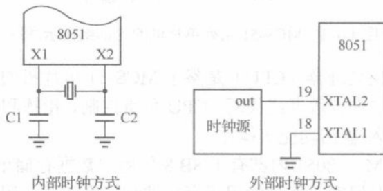
图 1-1-3 8051 单片机的时钟电路
