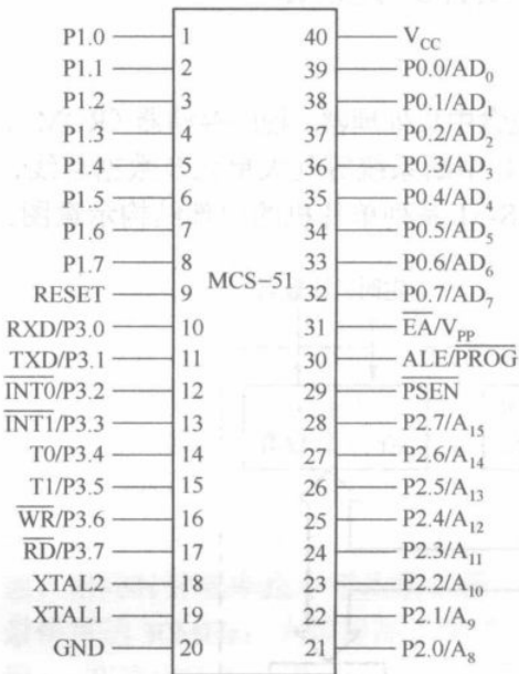
图 1-1-2 MCS-51 单片机的引脚分布
