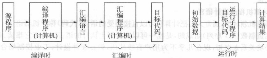
(b) 分为三个阶段的编译过程
