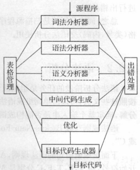
图 1.3 编译阶段
