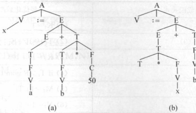
图 1.4 语法树
