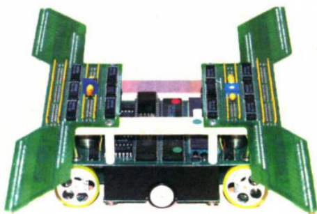
图1-1-3 1991年第12届全日本 Micromouse国际公开赛参赛鼠
