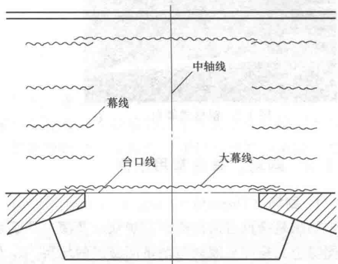
图 1-4 镜框式主舞台术语说明
