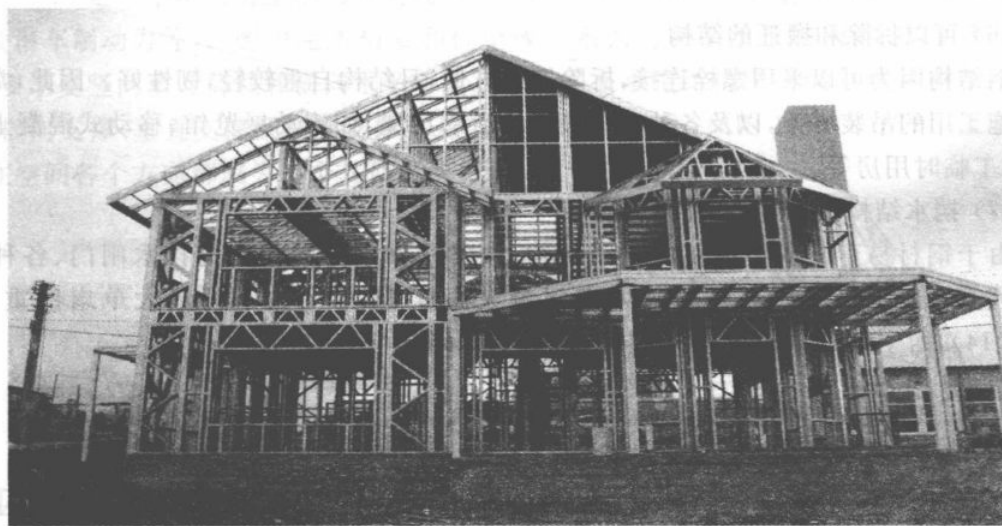
图 1.11 冷弯薄壁型钢结构
