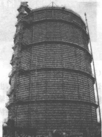
图 1.15 西宁特钢煤气柜
