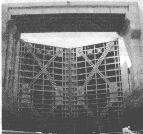
图 1.14 三峡船闸人字门
