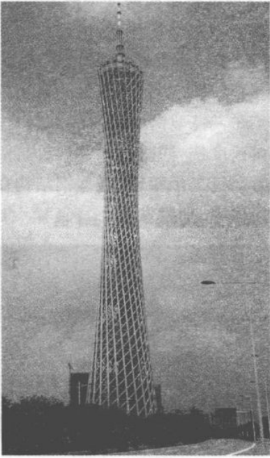
图 1.12 广州新电视塔
