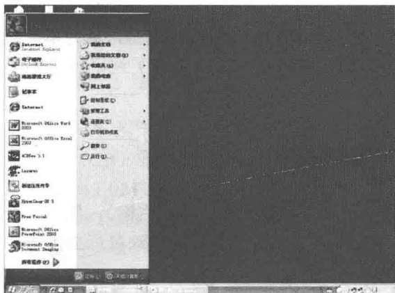
图 1-5 “开始”菜单
