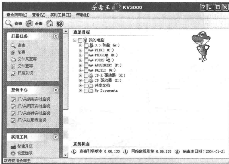
图 1-11 KV3000 窗口
