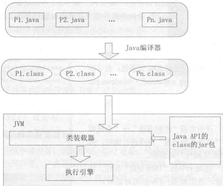
图 1-7 Java 程序运行环境
