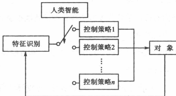
图 1-5 仿人控制的结构图
