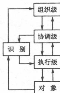
图 1-2 分级递阶智能控制结构
