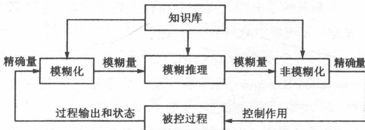
图 1-1 模糊控制系统的一般结构
