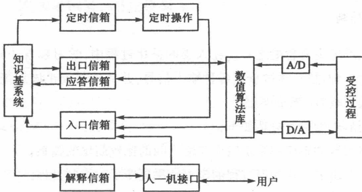
图 1-4 专家控制系统原理图
