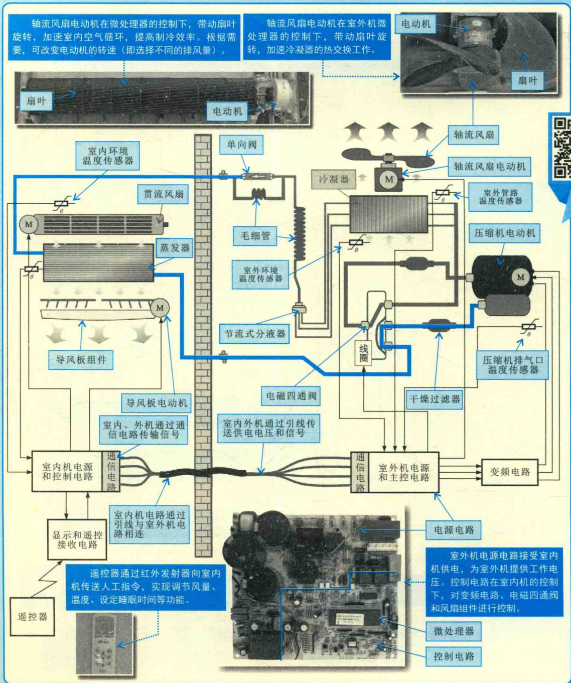
【空调器的电气控制过程】
