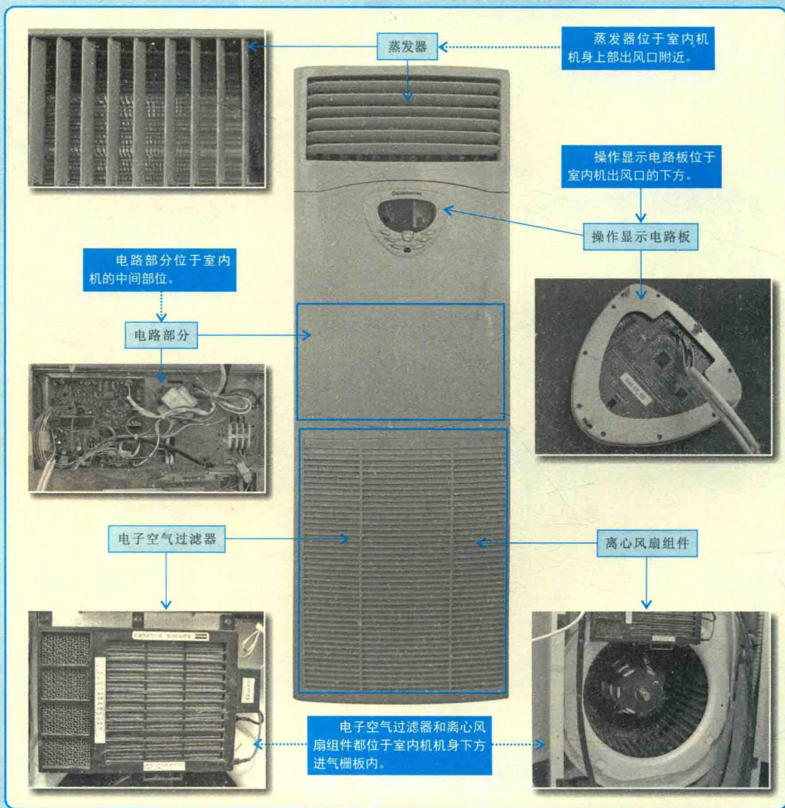
【分体柜式空调器室内机的结构】
