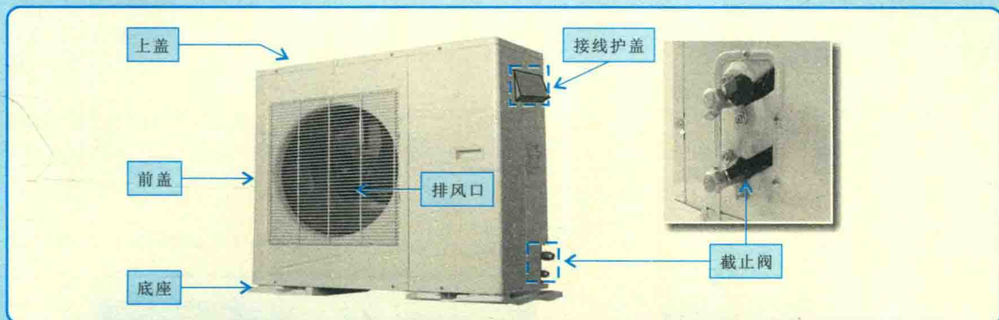
【变频空调器室外机的外部结构】
