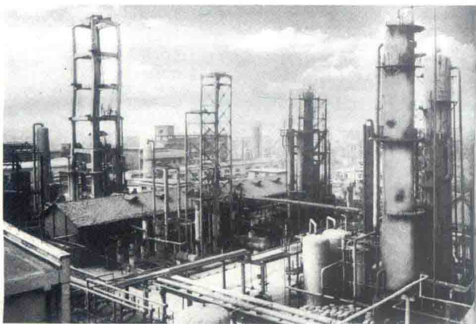
◀ 上世纪七十年 代攸县荣获全 国“五小工业” 先进县。图为 上世纪七十年 代攸县氮肥厂 造气厂区一角
