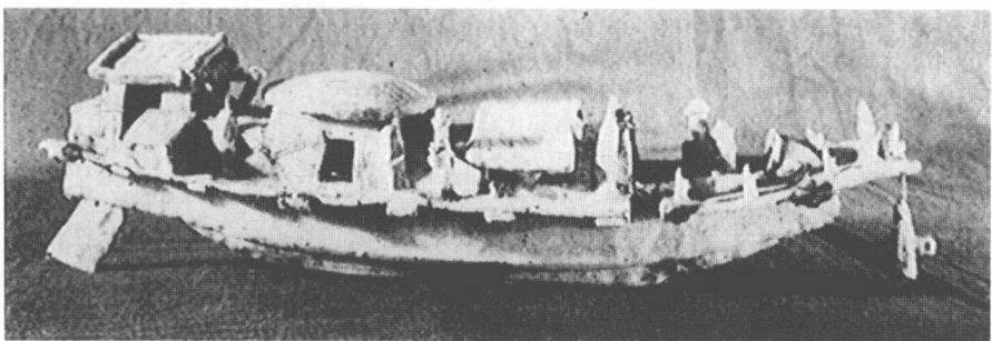
插图 13. 公元 1 世纪的广州墓穴出土的汉代陶船模型；这是所有文化中已知最早的艄柱舵例证。
