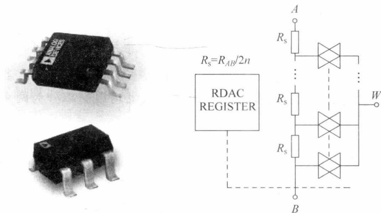
图 1.8 数字电位器的外形与内部结构
