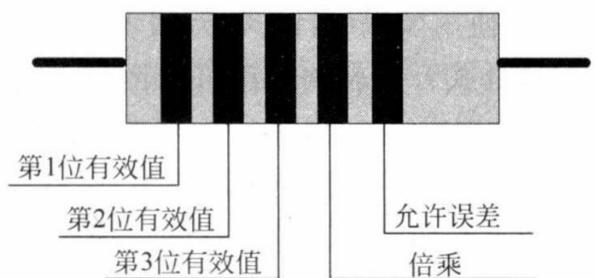
图 1.1 五道色环电阻示意图
