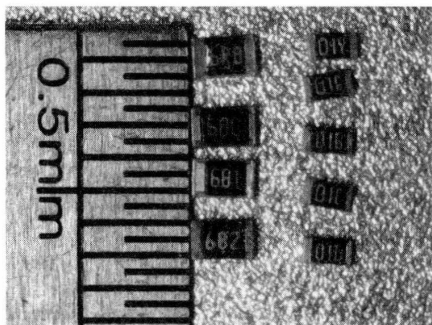
图 1.5 贴片电阻外形
